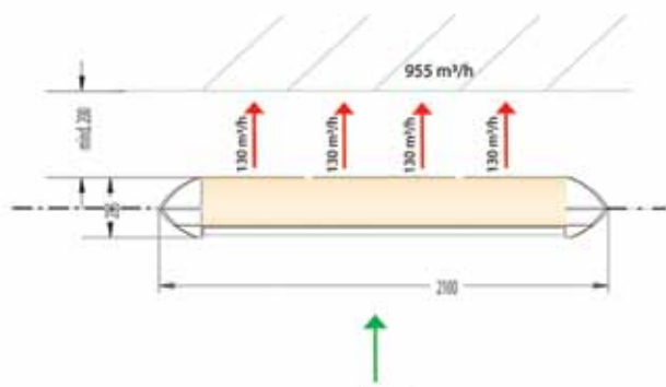
Rys. Schemat przepływu powietrza
